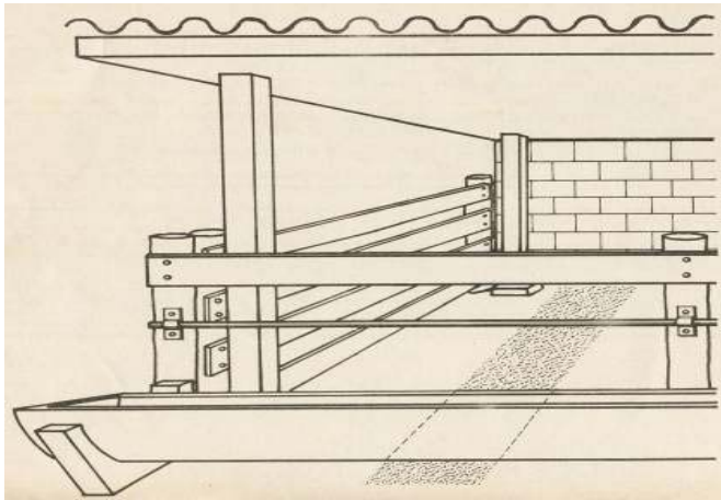
Gambar 18. Kandang pembesaran tampak dari depan
