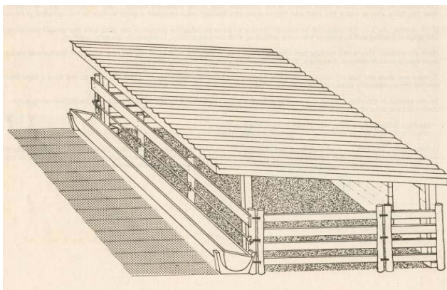
Gambar 11. Kandang kelompok beratap seluruhnya
