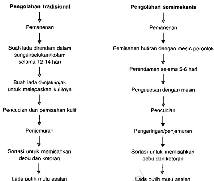
Gambar 2. Tahapan pengolahan lada putih secara tradisional dan semi mekanis.
