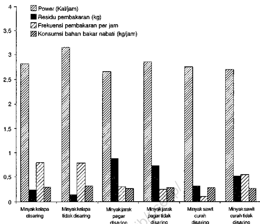
Gambar 7. Kinerja kompor tekan menggunakan beberapa jenis bahan bakar nabati.
