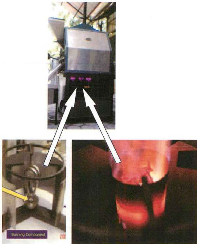
Gambar 8. Mesin penyangrai kopi menggunakan kompor berbahan bakar nabati asal minyak jarak pagar.
