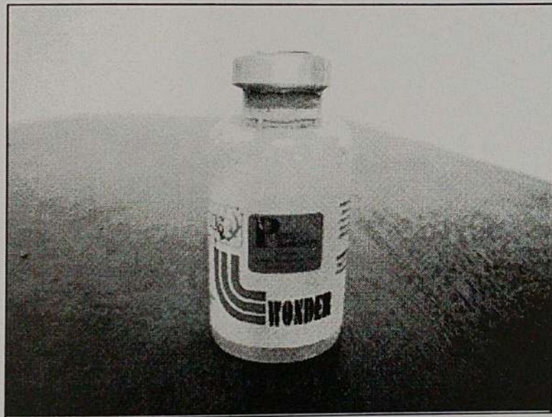
Progesteron
