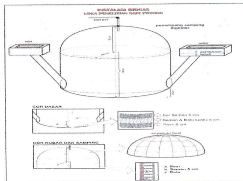
Gambar 21. Diagram Biogas Lolitsapi
