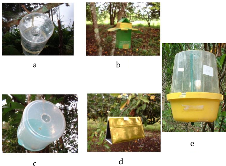
Gambar 19. Beberapa model perangkap lalat buah: (a) botol bekas air mineral, (b) modifikasi perangkap gypsy moth , (c) perangkap steiner, (d) perangkap delta transparan, dan (e) perangkap McPhail.
