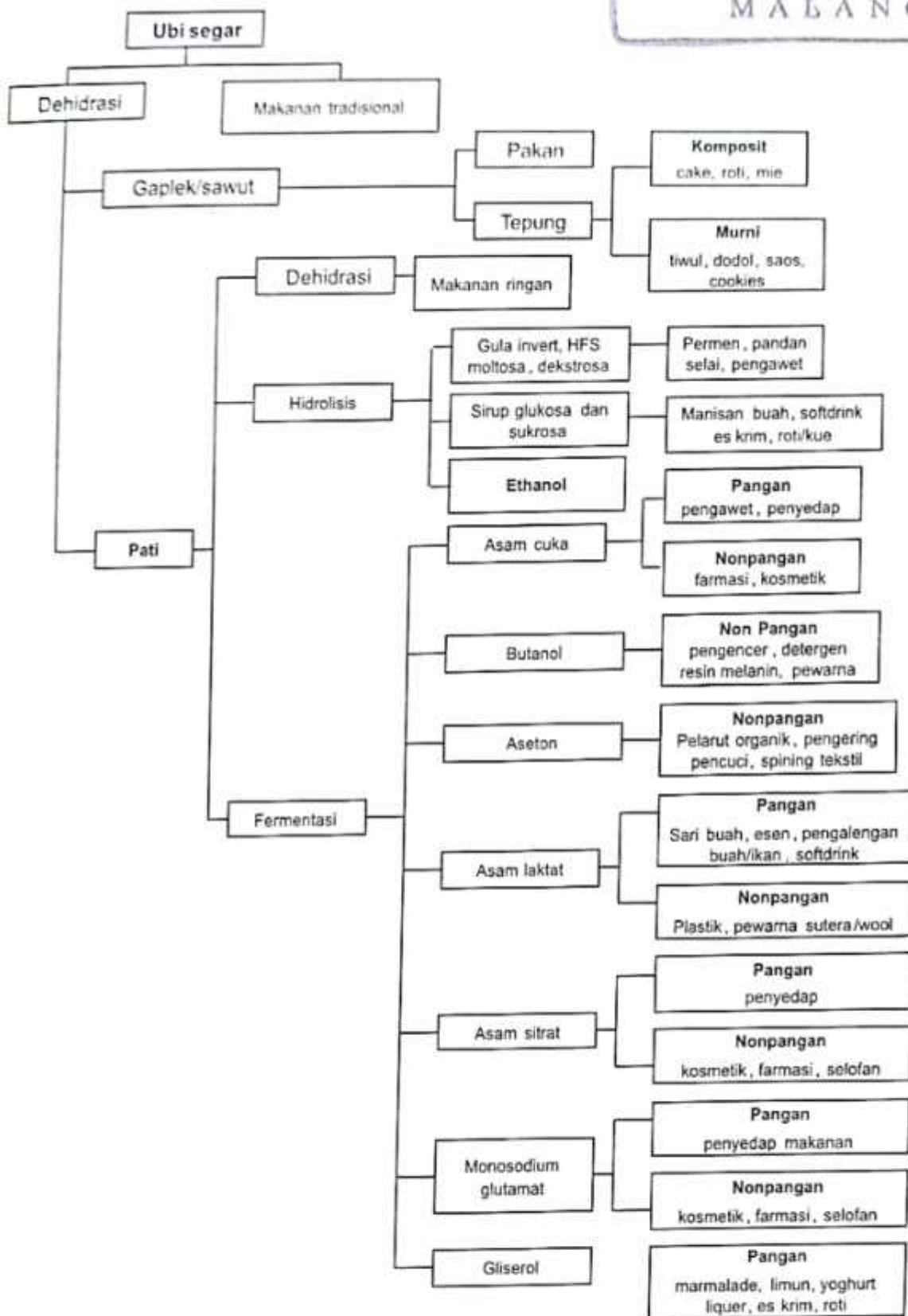
Gambar 2.2. Diagram alir industri hulu dan hilir multiproduk.
