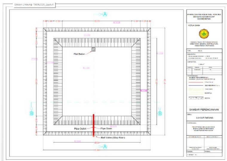
Gambar 3. Desain embung berlapis geomembran pada lahan Food Estate Hortikultura 200 ha di Kabupaten Humbang Hasundutan, Provinsi Sumatra Utara.
