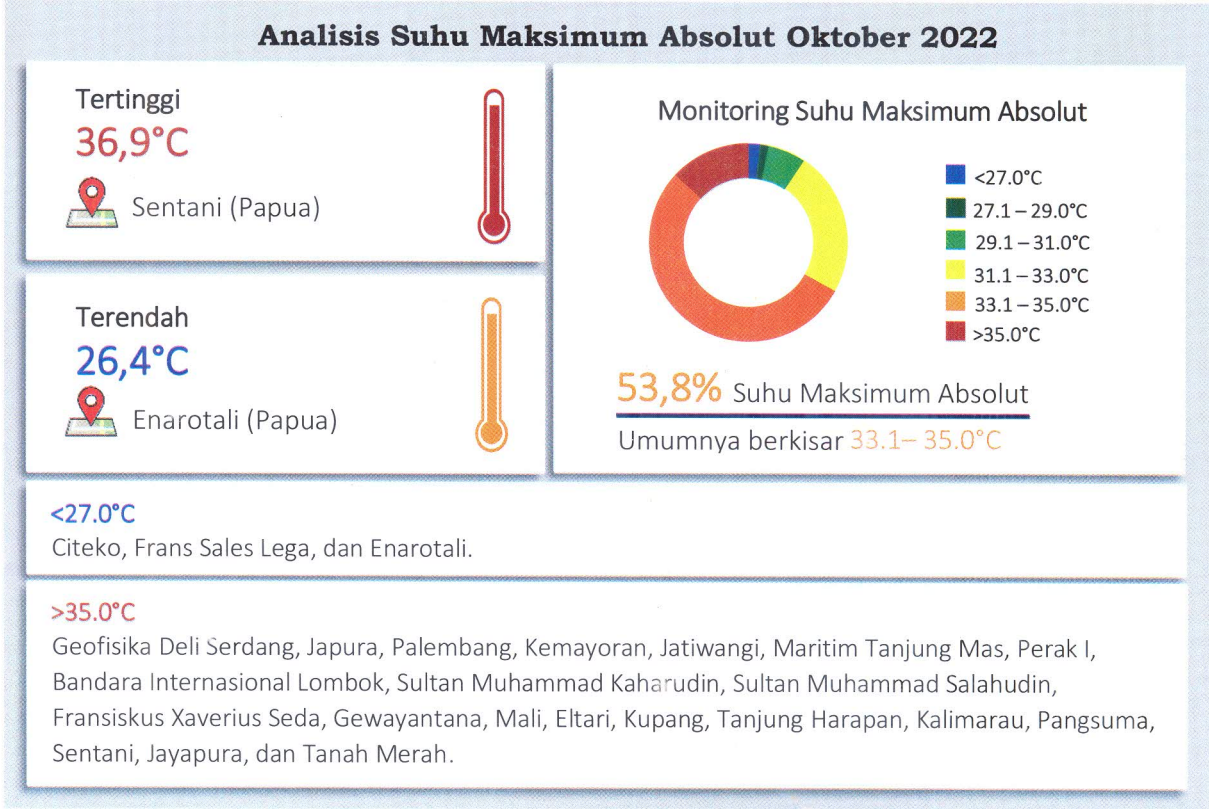
Gambar 1.3 Monitoring Suhu Udara Maksimum Absolut Oktober 2022
