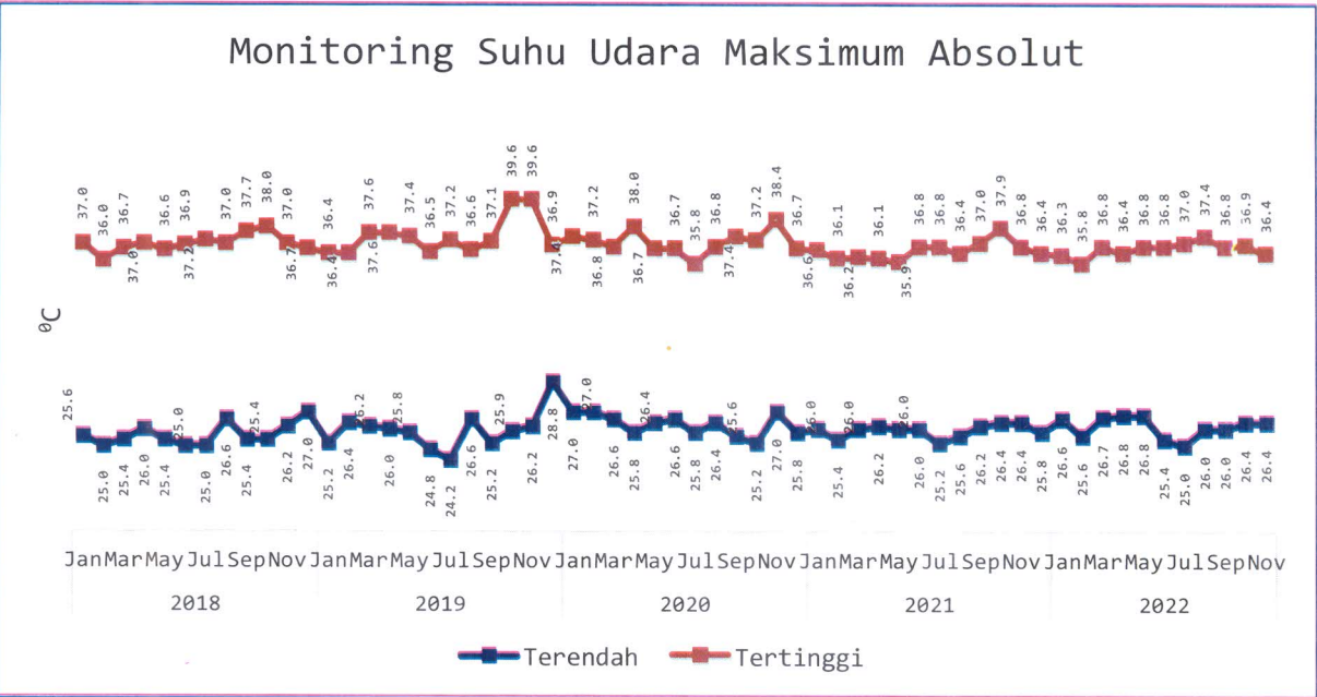
Gambar 1.1 Monitoring Suhu Udara Maksimum Absolut Tertinggi dan Terendah Januari 2018 - November 2022
