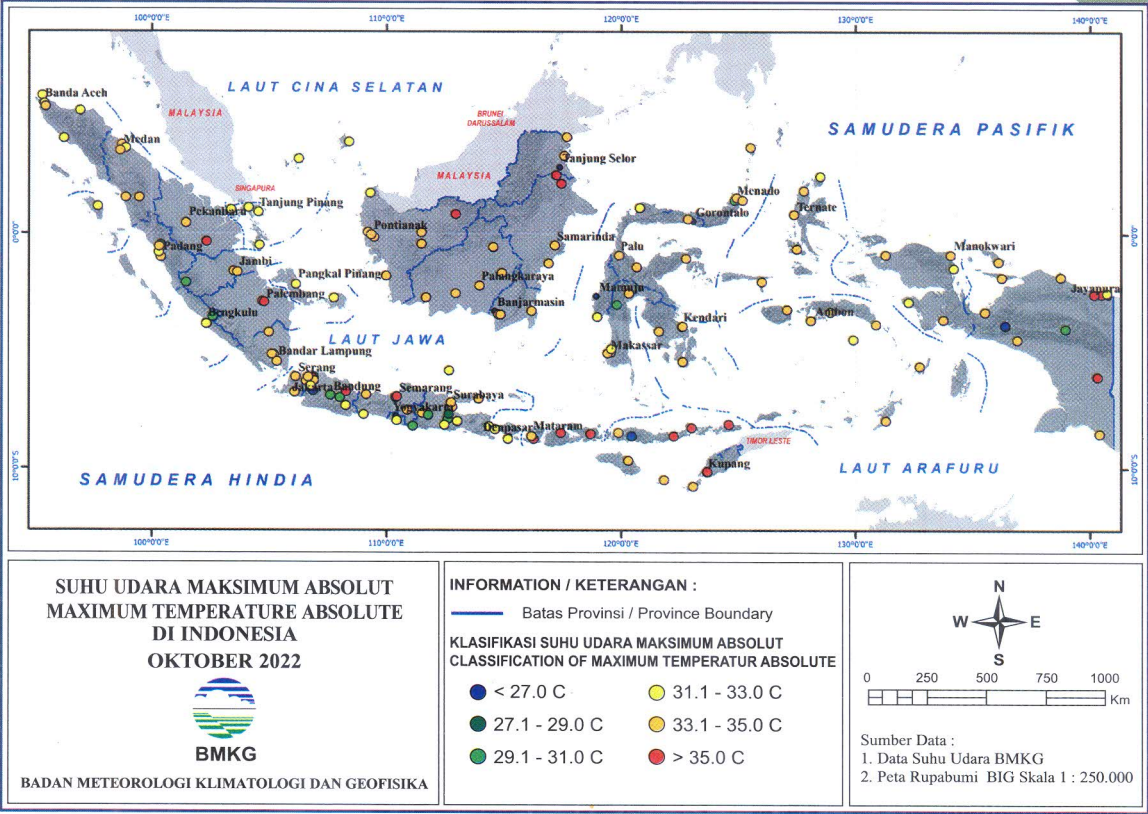
Gambar 1.3 Monitoring Suhu Udara Maksimum Absolut Oktober 2022
