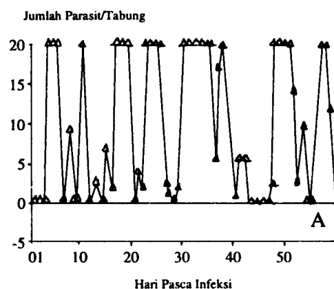
Gambar 1A. Fluktuasi jumlah parasit dalam darah seekor kerbau dewasa yang diinfeksi dengan T. evansi
